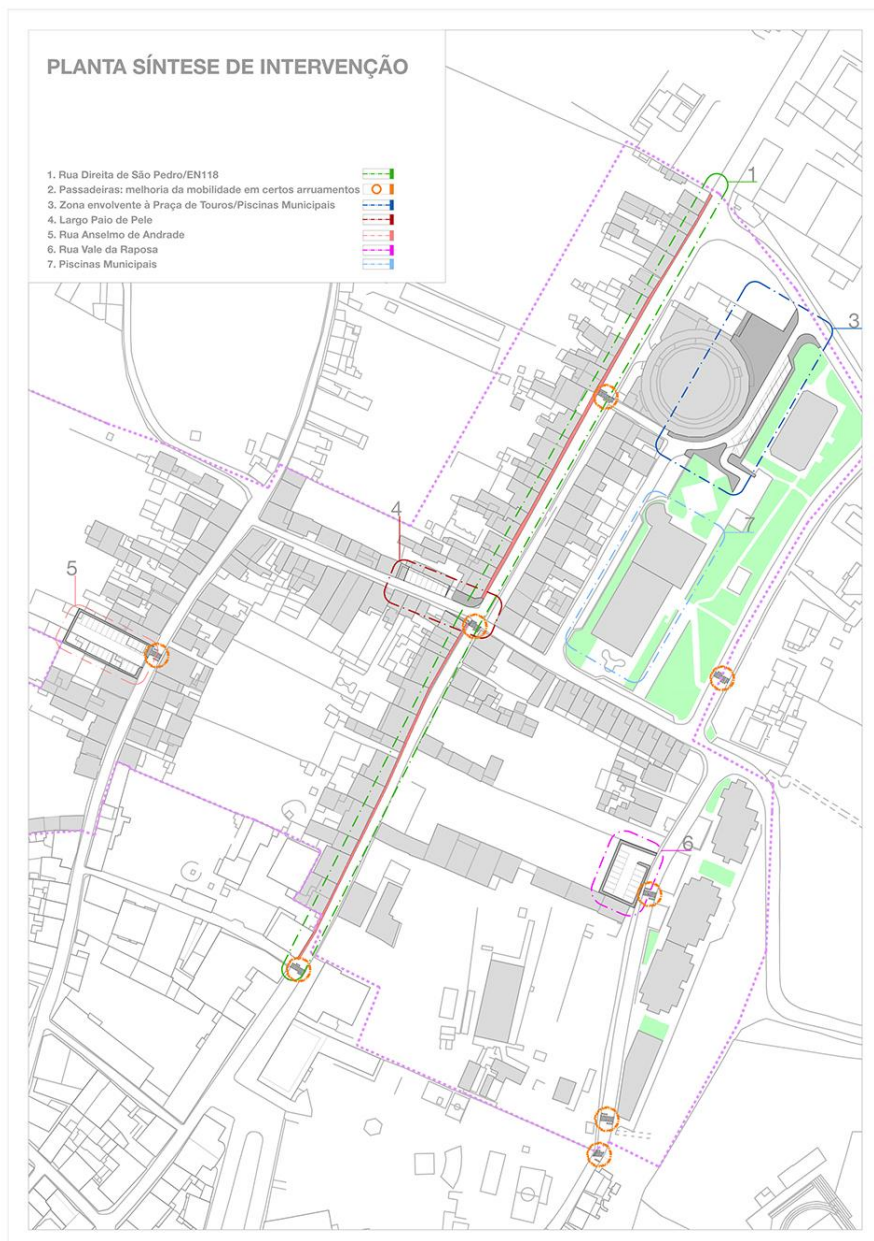
Planta 16: Planta síntese de intervenção
