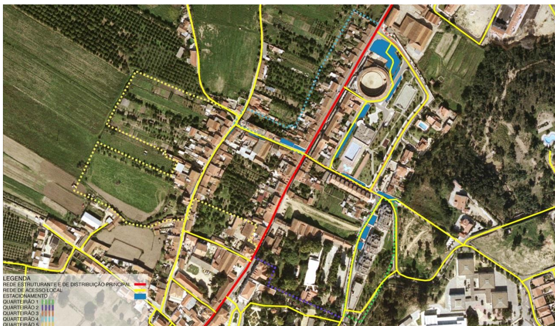
Planta 14: Estacionamento e hierarquia viária
